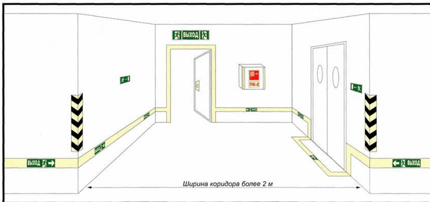
Рисунок Б.1 - Пример обозначения элементами ФЭС коридора.
