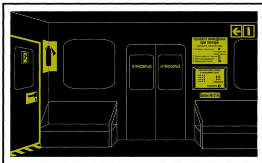
Рисунок Б.8 - Пример обустройства элементами ФЭС вагона электропоезда метрополитена после отключения освещения
