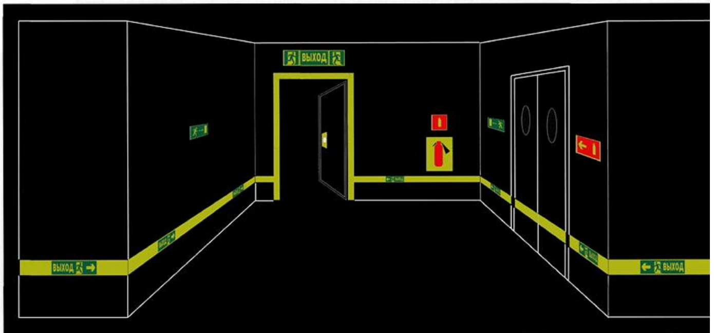
Рисунок Б.3 - Пример вида коридора с элементами ФЭС после отключения освещения
