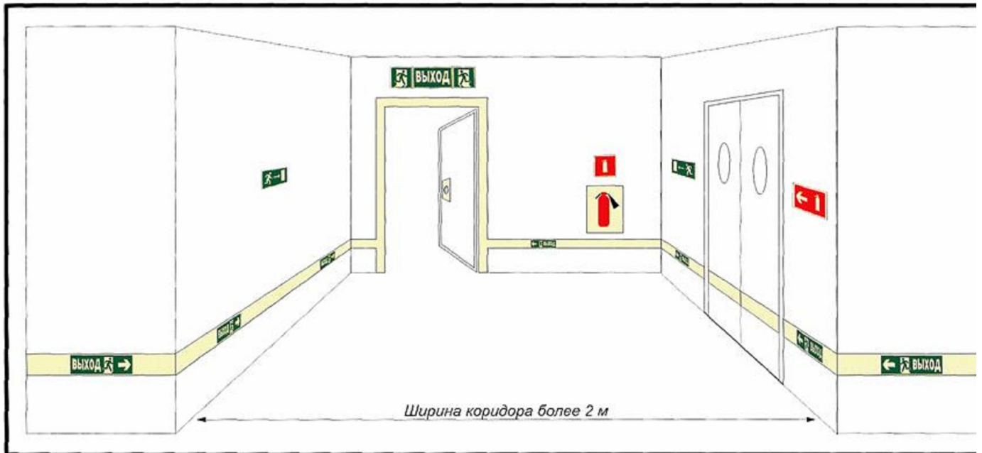
Рисунок Б.2 - Пример обозначения элементами ФЭС коридора.
